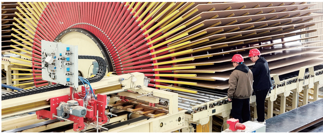
工人在山东省临沂市平邑县一家木业企业板材生产线上工作(2026年3月16日摄)。(新华社发)
